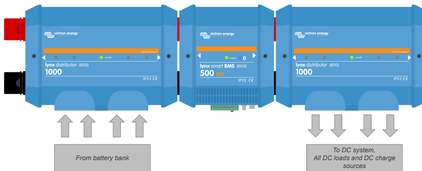
Exemple d'orientation d'un module Lynx : les batteries se connectent à gauche et tous les consommateurs et les chargeurs se connectent au côté droit
