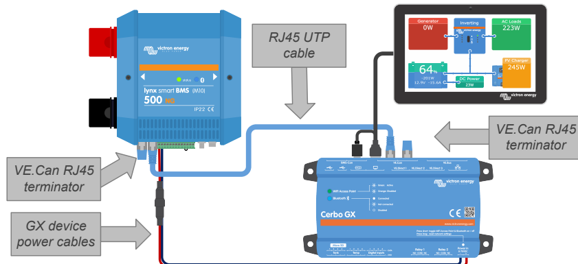
Exemple de câblage entre Lynx Smart BMS NG et un Cerbo GX avec GX Touch
