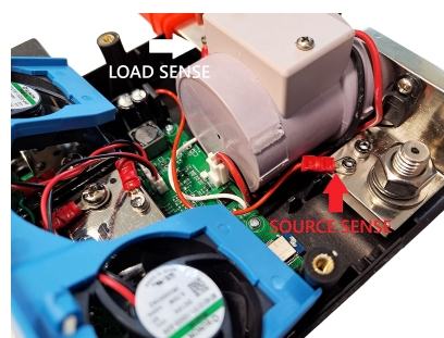
Fils permutés pour distribution électrique inversée
