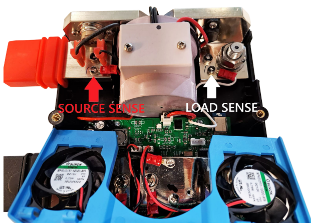
Détection de la tension source et consommateur
