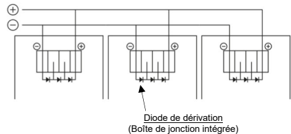
Schéma 2. Parallèle pour plus de courant
