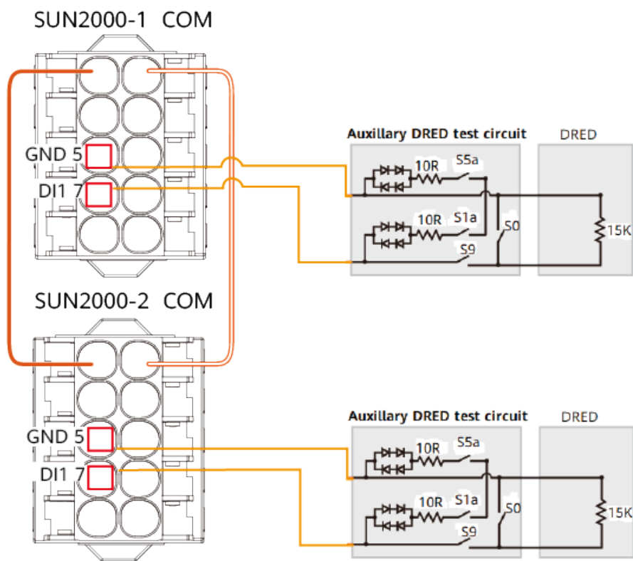
Figure 7-7 Schéma de câblage pour la fonction DRM
