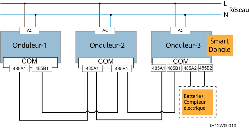
Figure 5-14 Mise en réseau du Smart Dongle (les composants dans l'encadré en pointillé sont facultatifs)
