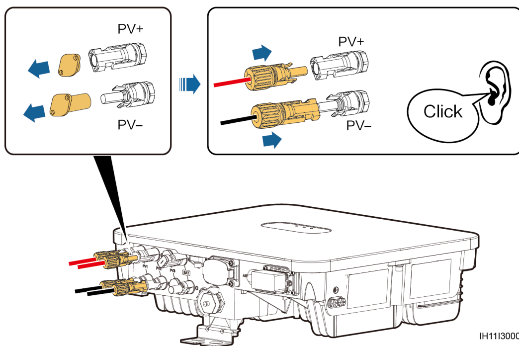
Figure 5-10 Connexion des câbles d'alimentation d'entrée CC
