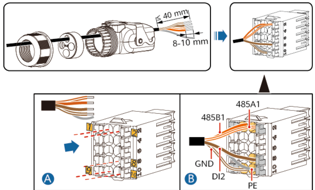
Figure 5-25 Installation du câble (connexion au SmartGuard)
