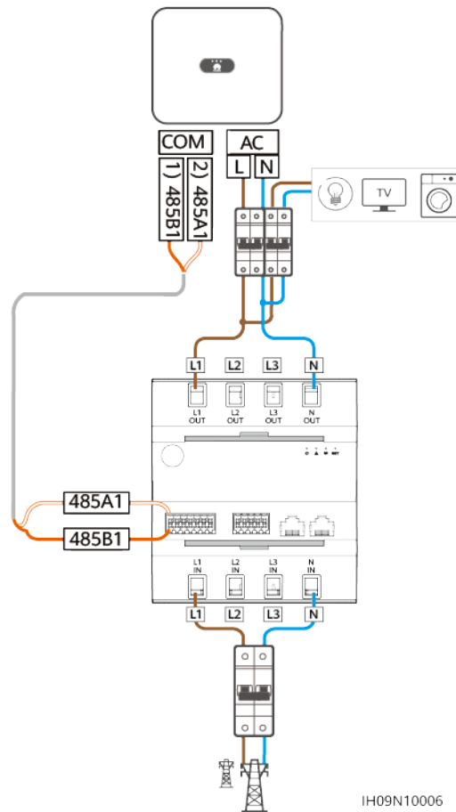
Figure 5-20 Connexion des câbles à l'EMMA
