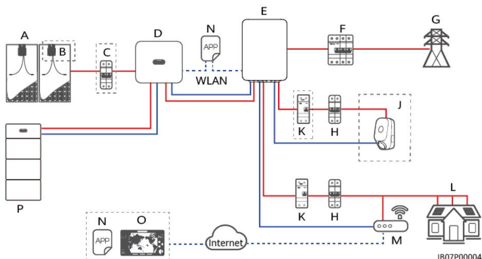
Figure 2-4 Mise en réseau du SmartGuard (les composants dans les encadrés en pointillés sont facultatifs)
