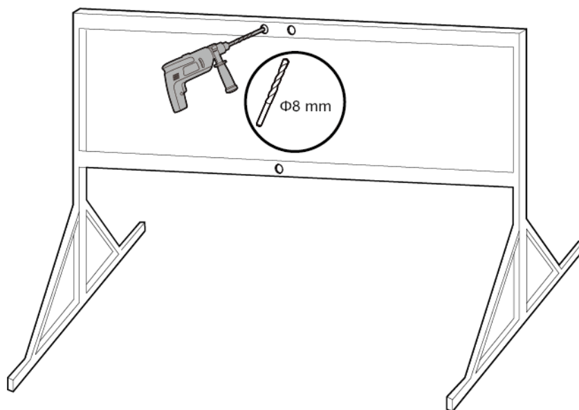
Figure 4-12 Perçage des trous
