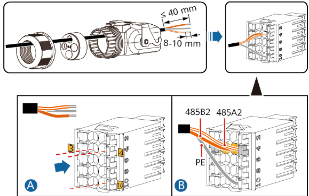
Figure 5-29 Installation du câble (connexion au compteur électrique)
