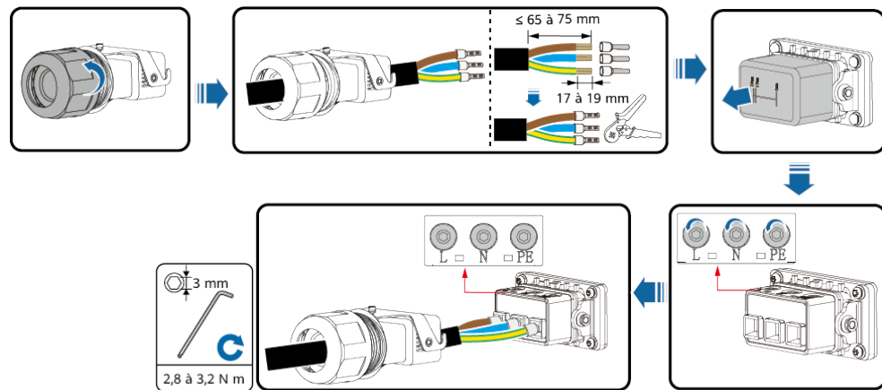
Figure 5-4 Installation du câble d'alimentation CA
