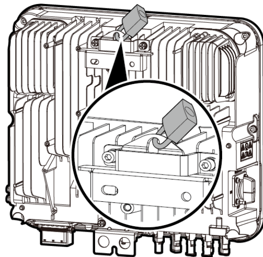
Figure 4-15 Installation d'un cadenas antivol
