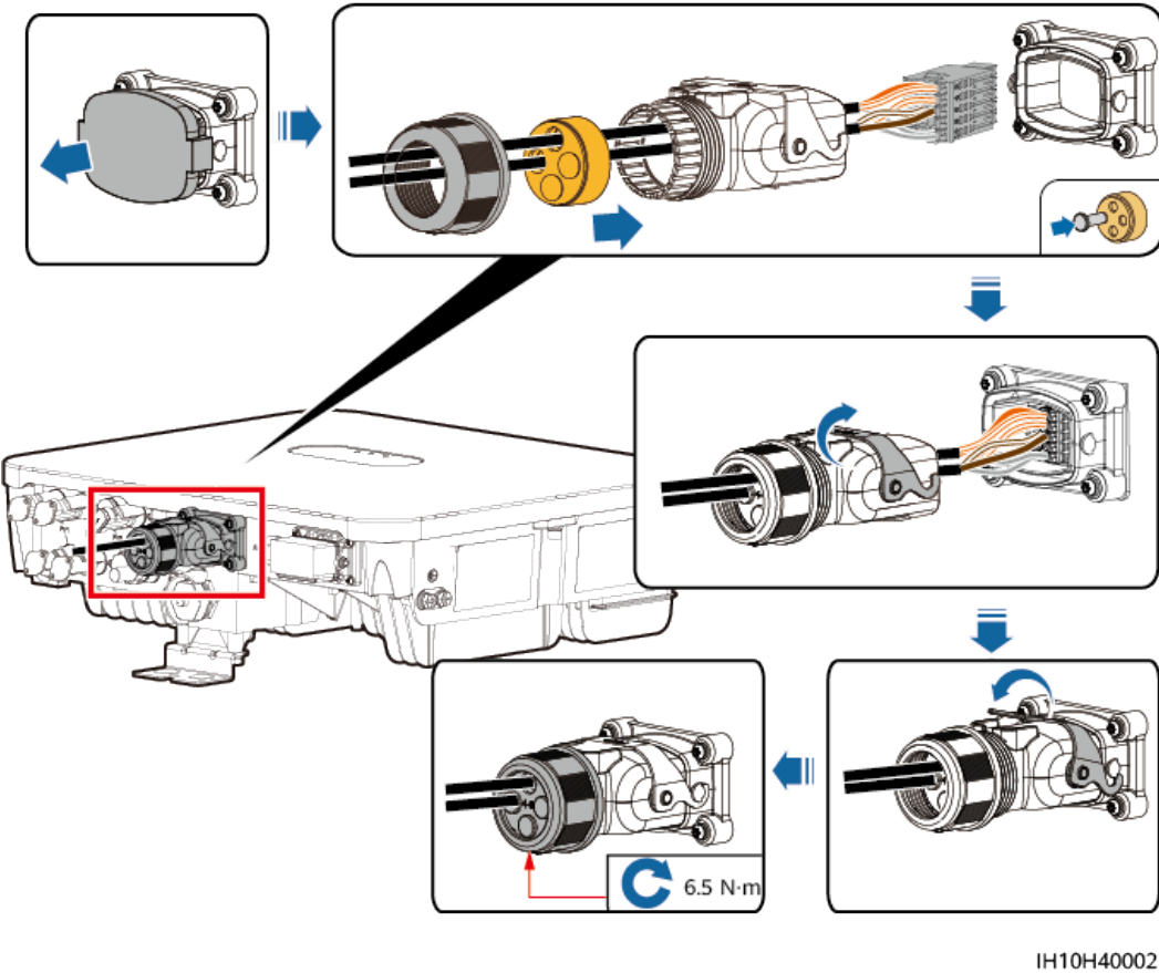
Figure 5-23 Fixation du connecteur du câble de signal
