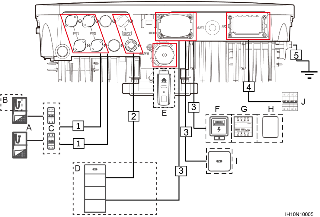
Figure 5-1 Connexions des câbles de l'onduleur (les composants dans l'encadré en pointillé sont facultatifs)
