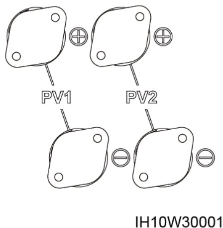
Figure 5-7 Bornes d'entrée CC
