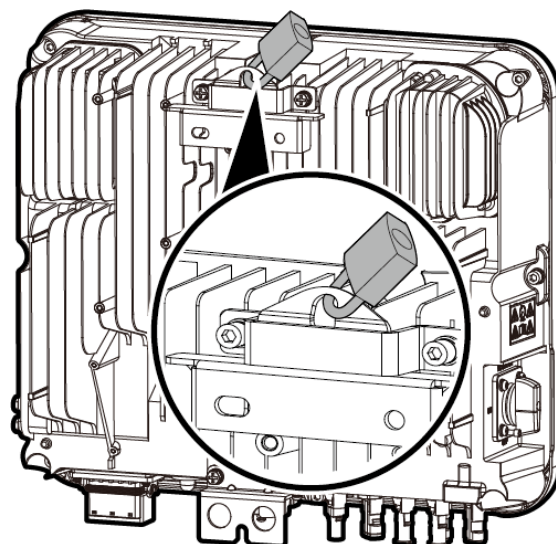
Figure 4-10 Installation d'un cadenas antivol
